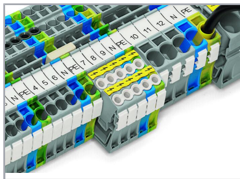
Réducteur isolant de sécurité (2002-171) et obturateur de protection (2002-115)
