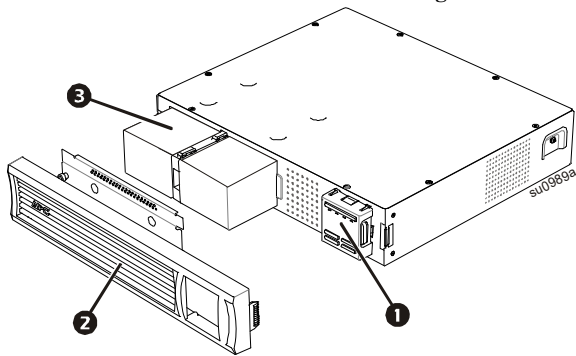
SMT1000RM2UC, SMT1000RMI2UC, SMT1500RM2UC et SMT1500RMI2UC Montage en baie
