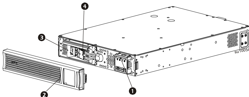
SMT2200RM2UC, SMT2200RMI2UC, SMT3000RM2UC et SMT3000RMI2UC Montage en baie
