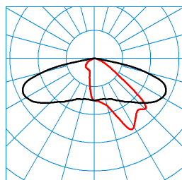
Jovie 50-AB2L-LRA/4200-730 4G1 ET (CLO end value) TX301177 ■ C0 - C180 ■ C90 - C270 DIN 5040: A30 UTE: 1,00 G CEN Flux Code: 34 71 96 100 100
