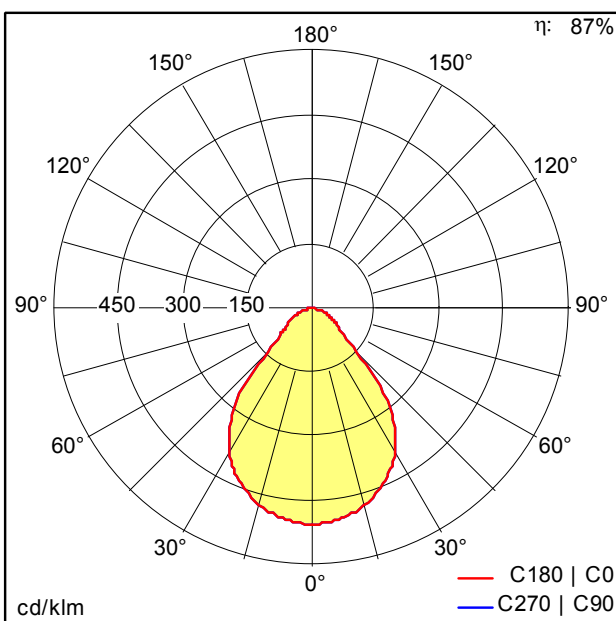
ST7983_N.Idt
