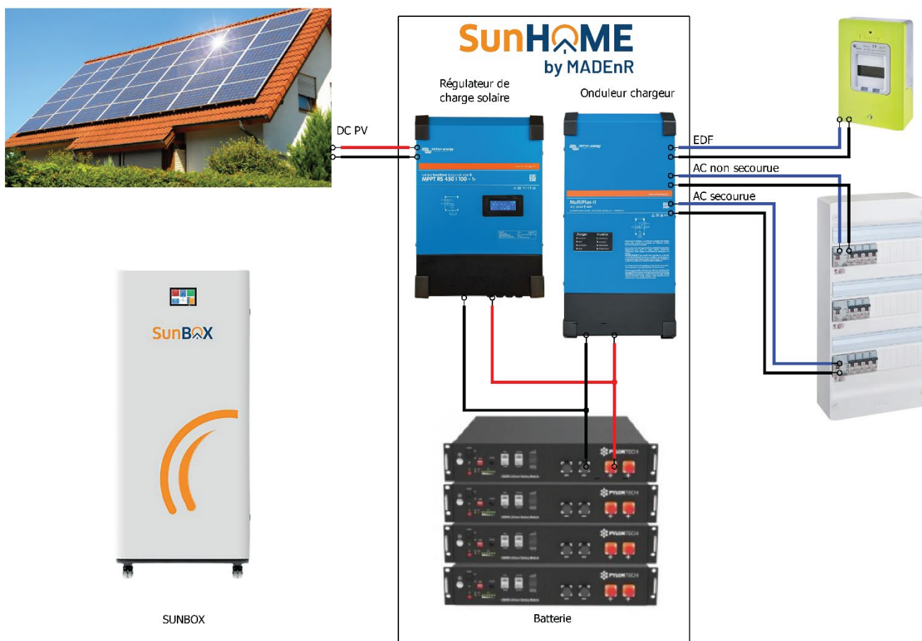
Figure 48 : Schéma de principe de la SunBox
