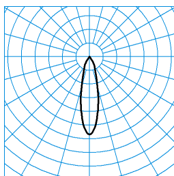
E-Line 7751 B.VEO RFS-MF 05 20-M J05 ETDD L37 03 ■ C0 - C180 TX095403
