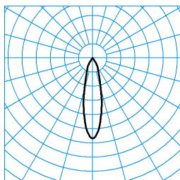
E-Line 7751 B.VEO RFS-MF-c 05 20-M J05 ETDD L37 03 ■ C0 - C180 TX095502
