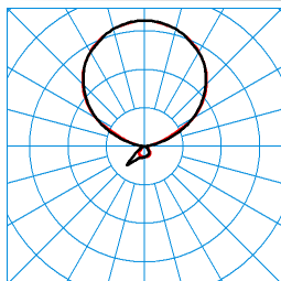
LuceoS S-U PAW-IL 300-830 05+LLWP(LEO1) TX245453 ■ C0 - C180 ■ C90 - C270 DIN 5040: E03 UTE: 0,08 D + 0,91 T CEN Flux Code: 53 86 96 8 100 49 82 98 92
