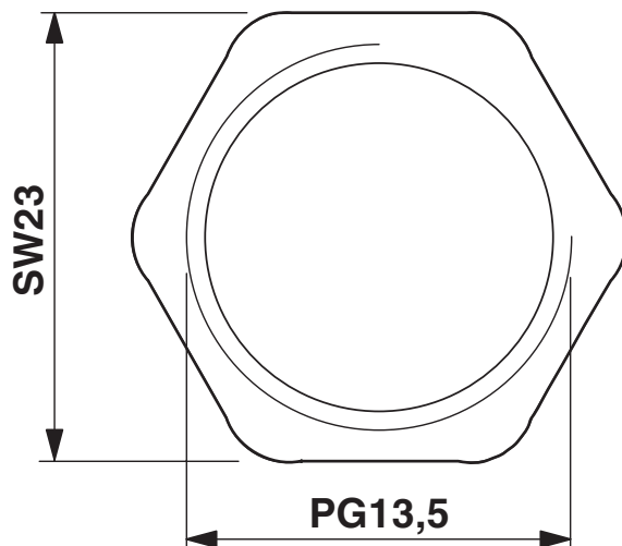
Dessin coté
