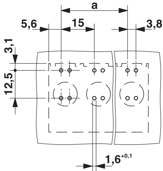
Dessin coté
