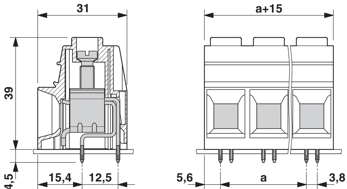
Dessin coté
