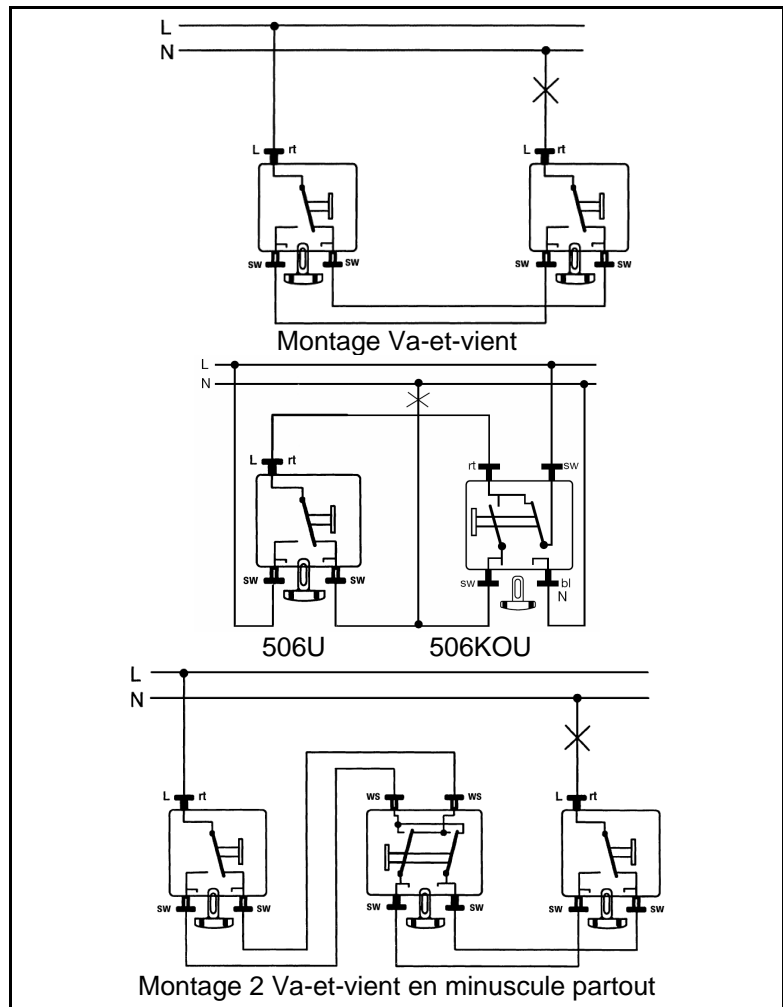
Schémas de raccordement 506 U
