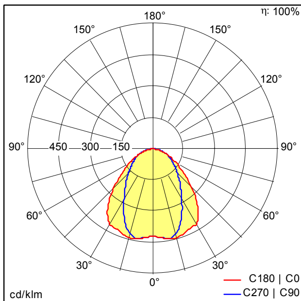
D44422AA_TEC_LED12000-865_L1500_VWB_LDE_SR_IP.idt
