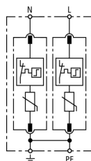
Schéma de principe du circuit DG M TN 275 NL
