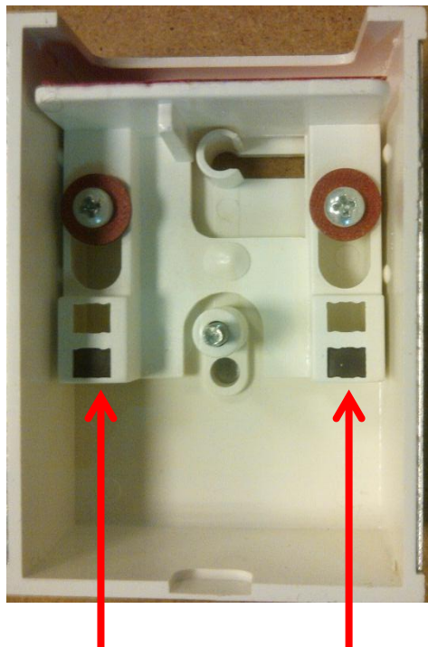
2 aimants qui actionnent les contacts magnétiques
