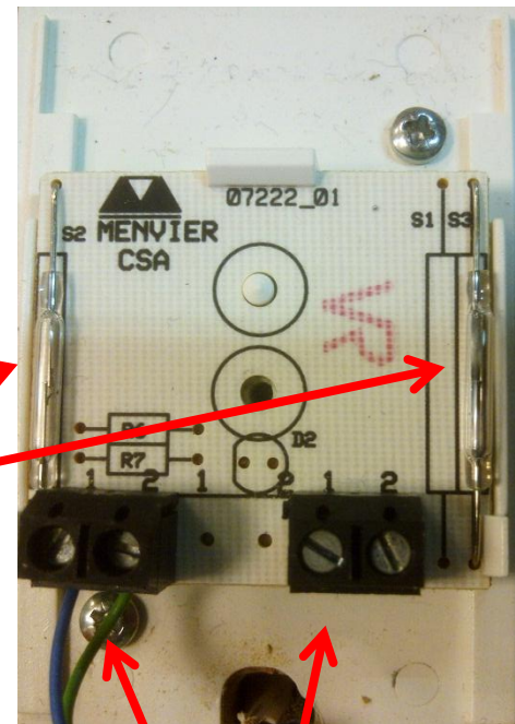
Intérieur du boîtier fixé
