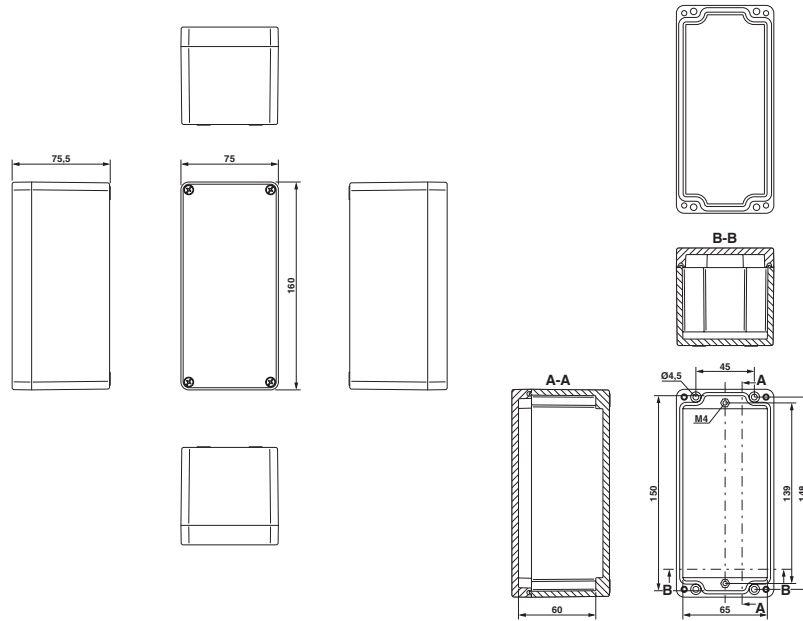
Dessin coté
