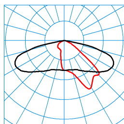
Jovie 50-AB2L-LRA/5100-730 6G1 ET (CLO initial value) TX300563 ■ C0 - C180 ■ C90 - C270 DIN 5040: A30 UTE: 1,00 G CEN Flux Code: 35 71 96 100 100
