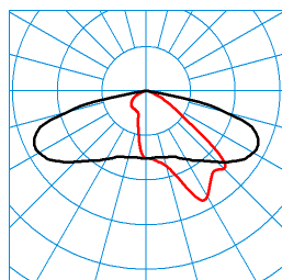
Jovie 50-AB2L-LRA/5100-730 6G1 ET (CLO end value) TX300958 ■ C0 - C180 ■ C90 - C270 DIN 5040: A30 UTE: 1,00 G CEN Flux Code: 35 71 96 100 100
