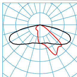
Jovie 50-AB2L-LRA/5100-730 6G1 ET TX068569 ■ C0 - C180 ■ C90 - C270 DIN 5040: A30 UTE: 1,00 G CEN Flux Code: 35 71 96 100 100
