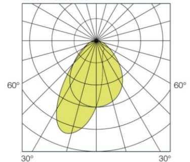
Fila 2 70 optique wallwasher code : 73367400
