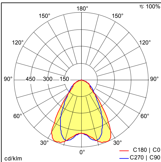
D44421AA_TEC_LED3700-865_L1000_WB_LDE_SR_IP.ltd
