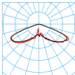
Publisca P1-RB6L-LR/2600-740 3G1S ET (CLO end value) TX300649
