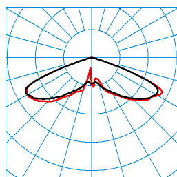
Publisca P1-RB6L-LR/2600-740 3G1S ET (CLO initial value) TX300917
