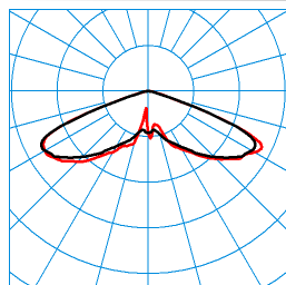
Publisca P1-RB6L-LR/2600-740 3G1S TX047635
