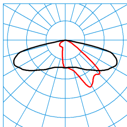
Jovie 50-AB2L-LRA/1000-730 2G1 ET (CLO initial value) TX300822 ■ C0 - C180 ■ C90 - C270 DIN 5040: A30 UTE: 0,98 l CEN Flux Code: 34 70 96 100 98
