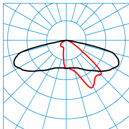
Jovie 50-AB2L-LRA/1000-730 2G1 ET (CLO end value) TX301155 ■ C0 - C180 ■ C90 - C270 DIN 5040: A30 UTE: 0,98 l CEN Flux Code: 34 70 96 100 98
