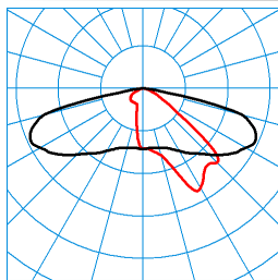
Jovie 50-AB2L-LRA/1000-730 2G1 ET TX068551 ■ C0 - C180 ■ C90 - C270 DIN 5040: A30 UTE: 0,98 l CEN Flux Code: 34 70 96 100 98
