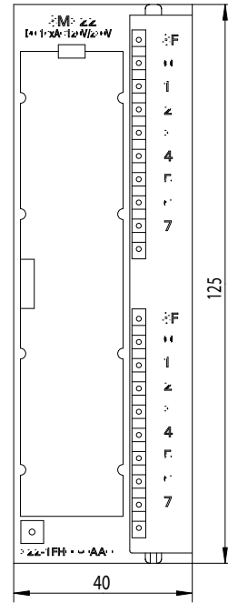
Vorne / Front
