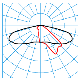
Jovie 50-AB2L-LR/1000-730 2G1 ET (CLO end value) TX300639 ■ C0 - C180 ■ C90 - C270 DIN 5040: A30 UTE: 0,98 l CEN Flux Code: 34 70 96 100 98
