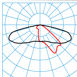
Jovie 50-AB2L-LR/1000-730 2G1 ET TX068531 ■ C0 - C180 ■ C90 - C270 DIN 5040: A30 UTE: 0,98 l CEN Flux Code: 34 70 96 100 98
