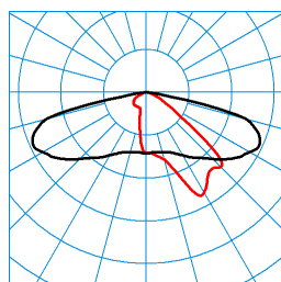
Jovie 50-AB2L-LR/1000-730 2G1 ET (CLO initial value) TX301256 ■ C0 - C180 ■ C90 - C270 DIN 5040: A30 UTE: 0,98 l CEN Flux Code: 34 70 96 100 98
