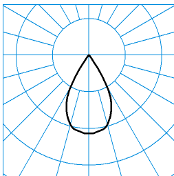
E-Line 7651 B.VEO RFS-VFL 05 20-M J05 ET L37 03 (150) ■ C0 - C180 TX124773
