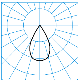
E-Line 7651 B.VEO RFS-VFL 05 20-M J05 ET L37 03 (225) ■ C0 - C180 TX124295
