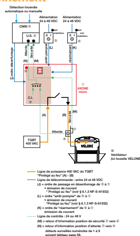
Schéma de principe d'un ventilateur 1 vitesse désenfumage.
