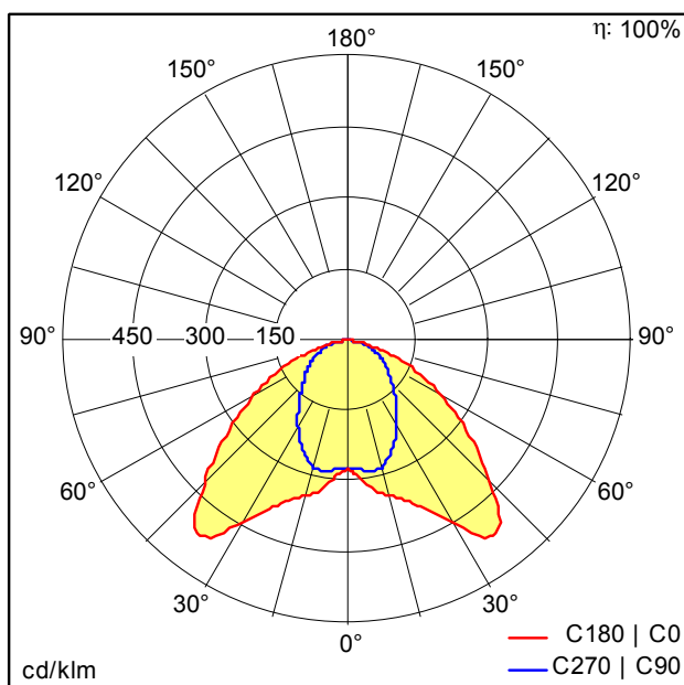
D41186AA_TECTON_C_LED8000-865_L1500_WSB_LDE_SR.Idt
