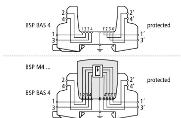
Schéma de principe du circuit avec et sans module
