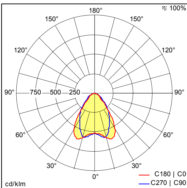
D35001AA_TECTON_C_LED3700-865_L1000_WB_LDE_WH.Idt
