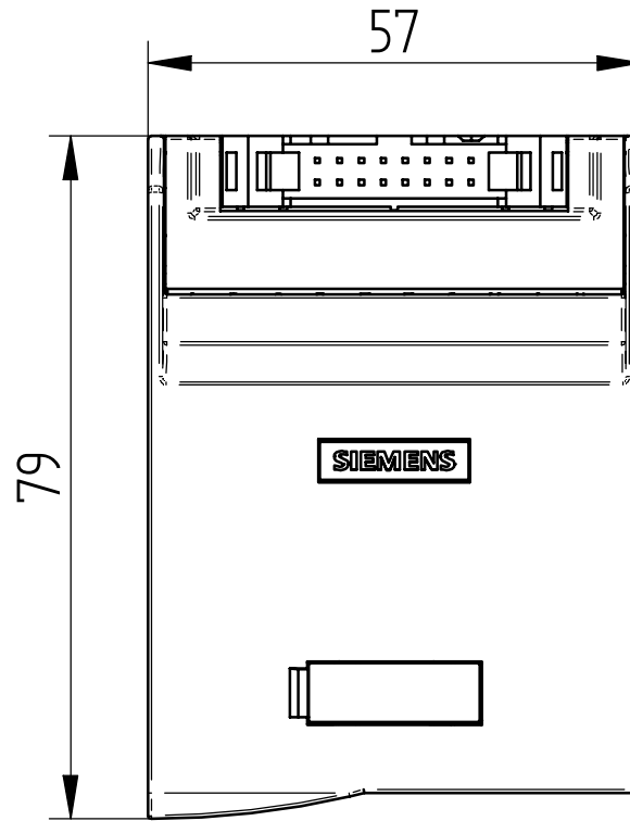
Vorne / Front
