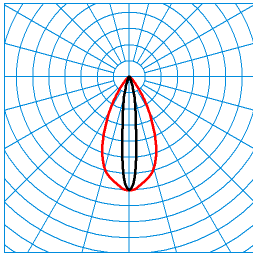
Altigo G2 C 60 SE6L/800-840 1G1P + G2 VE IP66 24V DC 30W TX113919 ■ C0 - C180 ■ C90 - C270 UGR I = 14,5 UGR q = 6,1 DIN 5040: A70 UTE: 1,00 A CEN Flux Code: 93 98 99 100 100
