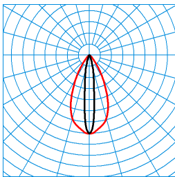
Altigo G2 C 60 SE6L/800-840 1G1P + G2 VE IP66 24V DC 80W TX113920 ■ C0 - C180 ■ C90 - C270 UGR I = 14,5 UGR q = 6,1 DIN 5040: A70 UTE: 1,00 A CEN Flux Code: 93 98 99 100 100
