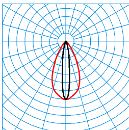
Altigo G2 C 60 SE6L/800-840 1G1P + VE IP66 24V DC 250W TX120505 ■ C0 - C180 ■ C90 - C270 UGR I = 14,5 UGR q = 6,1 DIN 5040: A70 UTE: 1,00 A CEN Flux Code: 93 98 99 100 100
