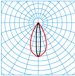
Altigo G2 C 60 SE6L/800-840 1G1P + G2 VE IP66 24V DC 240W TX113928 ■ C0 - C180 ■ C90 - C270 UGR I = 14,5 UGR q = 6,1 DIN 5040: A70 UTE: 1,00 A CEN Flux Code: 93 98 99 100 100
