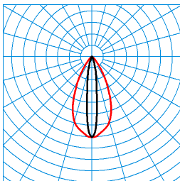
Altigo G2 C 60 SE6L/800-840 1G1P + VE IP66 24V DC 130W TX120438 ■ C0 - C180 ■ C90 - C270 UGR I = 14,5 UGR q = 6,1 DIN 5040: A70 UTE: 1,00 A CEN Flux Code: 93 98 99 100 100
