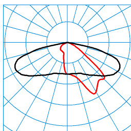
Jovie 50-AB2L-SLR1/6800-740 6G1 ET (CLO end value) TX301296 ■ C0 - C180 ■ C90 - C270 DIN 5040: A30 UTE: 1,00 G CEN Flux Code: 35 71 96 100 100
