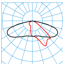
Jovie 50-AB2L-SLR1/6800-740 6G1 ET (CLO initial value) TX301568 ■ C0 - C180 ■ C90 - C270 DIN 5040: A30 UTE: 1,00 G CEN Flux Code: 35 71 96 100 100
