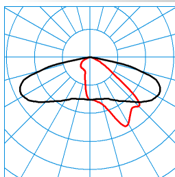
Jovie 50-AB2L-SLR1/6800-740 6G1 ET TX068575 ■ C0 - C180 ■ C90 - C270 DIN 5040: A30 UTE: 1,00 G CEN Flux Code: 35 71 96 100 100
