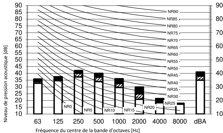
Mode rafraîchissement
