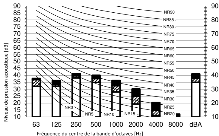
Mode chauffage
