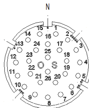
00008825 E-Part / Stift 26 polig
