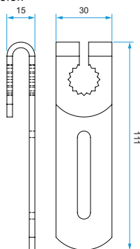
Dimensions poignée de commande CRGE / CRGN
