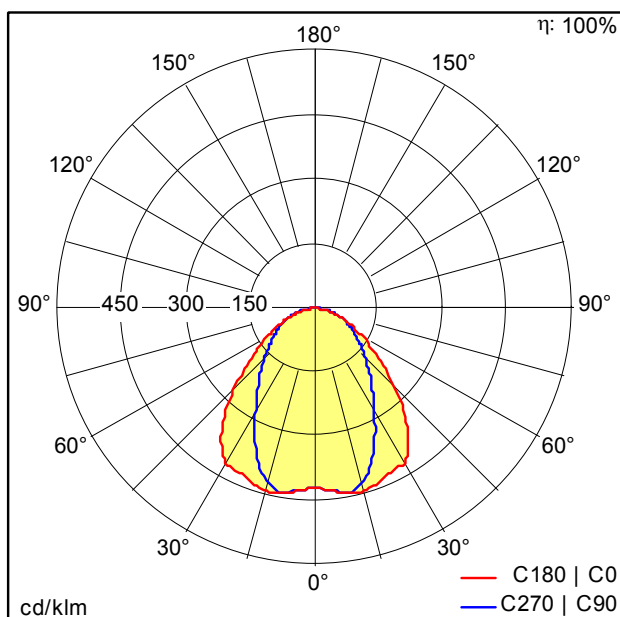
D44422AA_TEC_LED8000-865_L1000_VWB_LDE_SR_IP.idt
