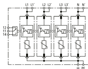
Schéma de principe du circuit DG MP TNS 275 FM
