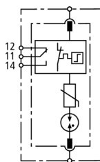
Schéma de principe du circuit DG S 385 VA FM
