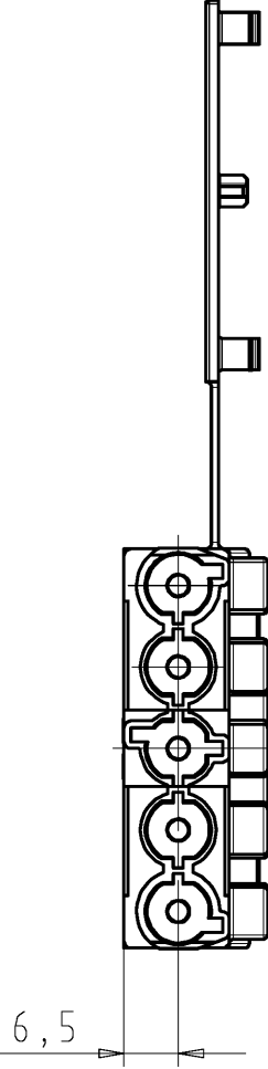
Darstellung M1:1 gezeichnet im montierten Zustand/ draw version in assembled state, scale 1:1
