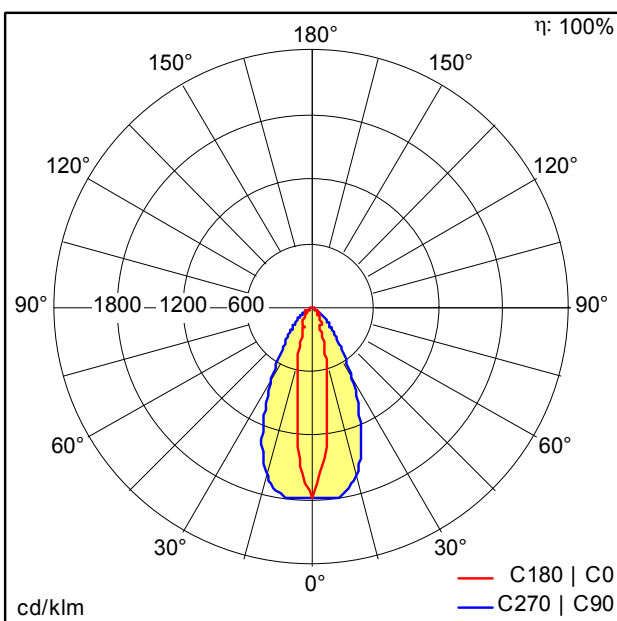
D34981_TECTON_C_LED8000_865_L1000_NB_EVG_WH.Idt
