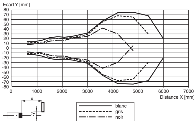
Courbe de réponse caractéristique (avec élimination de l'arrière-plan) LT(K)2-8-HS-6000
