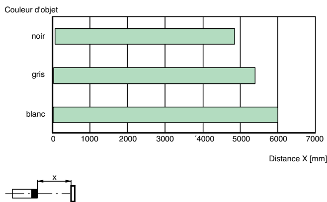
Domaines de détection avec élimination de l'arrière-plan LT(K)2-8-HS-6000
