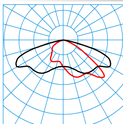
Jovie 70-AB7L-LRA/13500-730 12G1 ET TX068624 ■ C0 - C180 ■ C90 - C270 DIN 5040: A30 UTE: 1,00 G CEN Flux Code: 34 72 96 100 100
