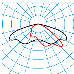
Jovie 70-AB7L-LRA/13500-730 12G1 ET (CLO end value) TX301437 ■ C0 - C180 ■ C90 - C270 DIN 5040: A30 UTE: 1,00 G CEN Flux Code: 34 72 96 100 100
