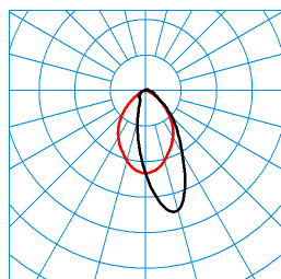
TX053252 DIN 5040: A50 UTE: 0,96 C + 0,04 T C0 - C180 C90 - C270
