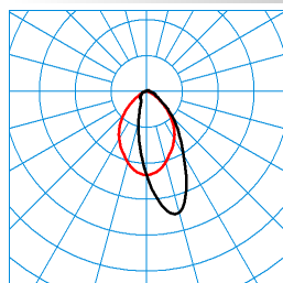
TX050713 DIN 5040: A50 UTE: 0,96 C + 0,04 T C0 - C180 C90 - C270
