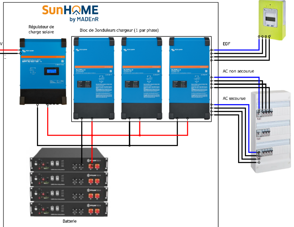
Figure 59 : Schéma de principe de la SunTri
