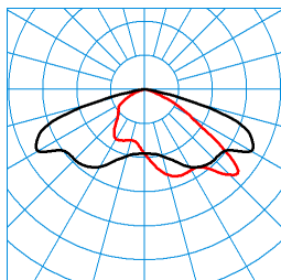
Jovie 70-AB7L-LR/20000-740 24G1 ET (CLO initial value) TX300554 ■ C0 - C180 ■ C90 - C270 DIN 5040: A30 UTE: 1,00 G CEN Flux Code: 35 73 97 100 100
