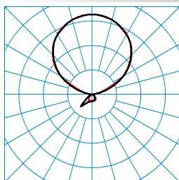
LuceoS S-U PAW-IL 300-840 05+LLWP(LEO1) TX245549 ■ C0 - C180 ■ C90 - C270 DIN 5040: E03 UTE: 0,08 D + 0,91 T CEN Flux Code: 53 86 96 8 100 49 82 98 92
