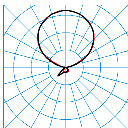
LuceoS S-U PAW-IL 300-840 05+LLWP(LEO2) TX245567 ■ C0 - C180 ■ C90 - C270 DIN 5040: E03 UTE: 0,08 D + 0,91 T CEN Flux Code: 53 86 96 8 100 49 82 98 92
