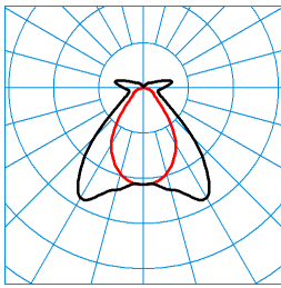
TugraHE Act 18 PW19 50 ETDD8 01 (ACTDSU) TX375150 ■ C0 - C180 ■ C90 - C270 DIN 5040: B41 UTE: 0,81 D + 0,19 T CEN Flux Code: 60 85 94 81 100 9 28 64 19
