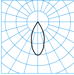
E-Line 7651 B.VEO RFS-WFL 05 20-M J05 ET L37 01 (225) TX123998 ■ C0 - C180 DIN 5040: A80 UTE: 0,82 A CEN Flux Code: 99 100 100 100 82
