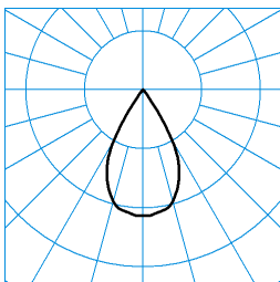
E-Line 7651 B.VEO RFS-VFL 05 20-M J05 ET L37 01 (225) TX124296 ■ C0 - C180 DIN 5040: A80 UTE: 0,82 A CEN Flux Code: 99 100 100 100 82
