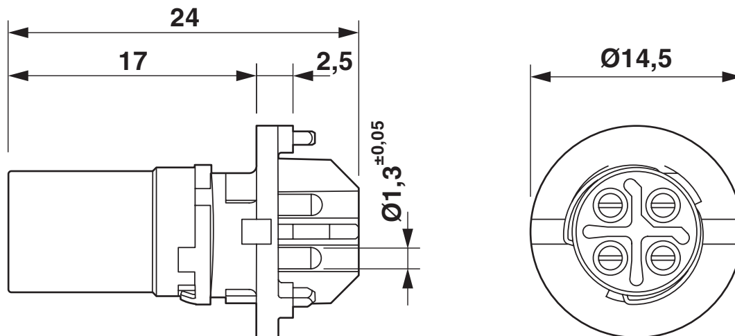
Dessin coté
