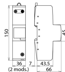
Dimensions DVCI 1 255
