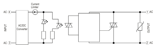
Contrôle AC/DC série GN+ Triac - 25 A
