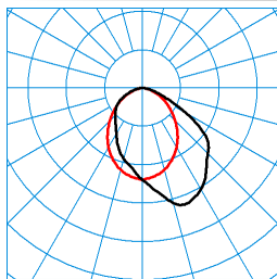
Opendo D2-L DW 52-840 ET 01 TX277472 ■ C0 - C180 ■ C90 - C270 DIN 5040: A40 UTE: 1,00 E CEN Flux Code: 50 83 97 100 100
