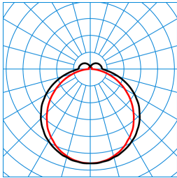
Olisq LWD3 DW 30-840 ET IP54 IK TX430035
